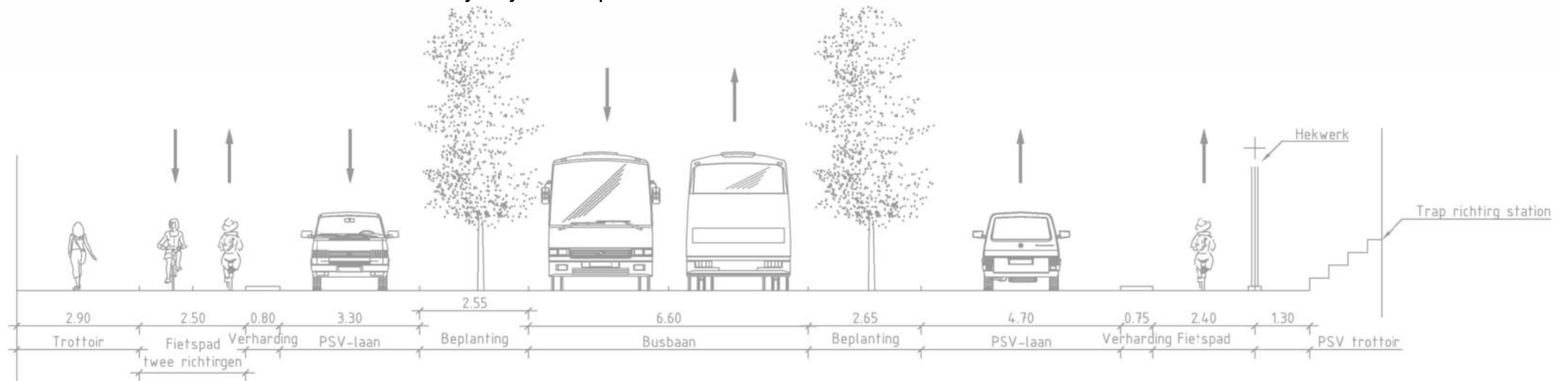
Bestaand dwarsprofiel PSV-laan
