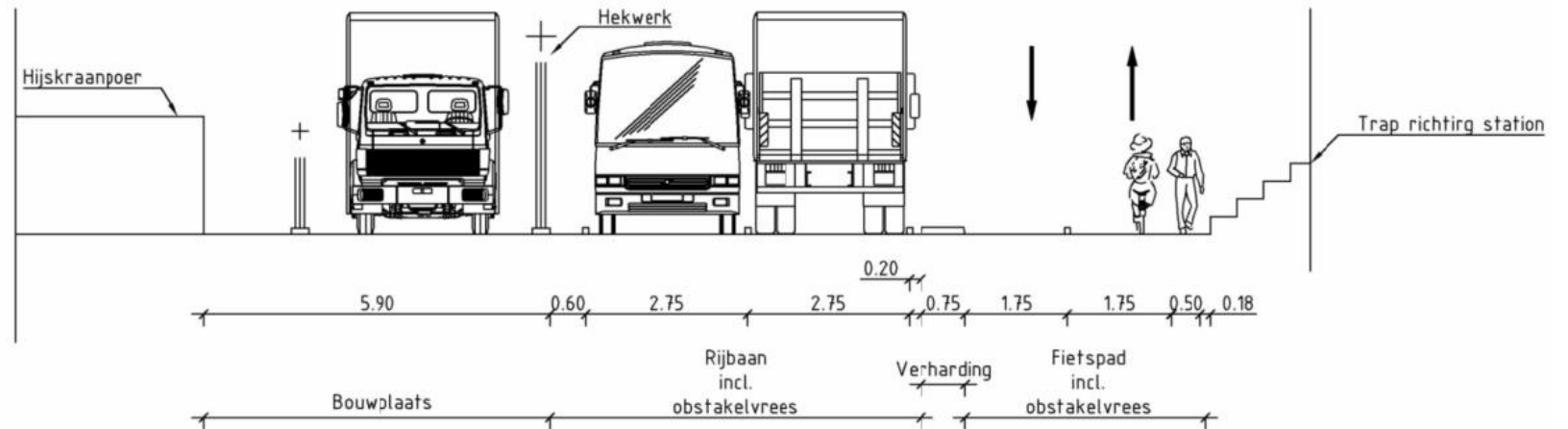
Tijdelijk dwarsprofiel PSV-laan
